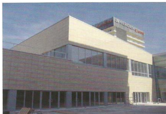
HOTEL "LAV" Split, keramičke ploče 67x 45 cm BWM potkonstrukcija ATK 100KL
