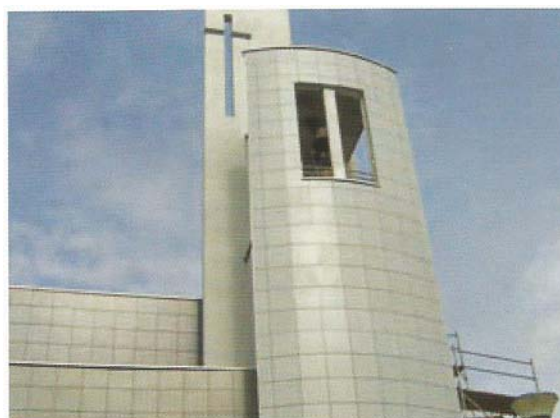
CRKVA SV. ČIRILA I METODA, Osijek - Divaltova ulica Keramičke ploče 60x60 cm na BWM potkonstrukciji ATK 100KL
